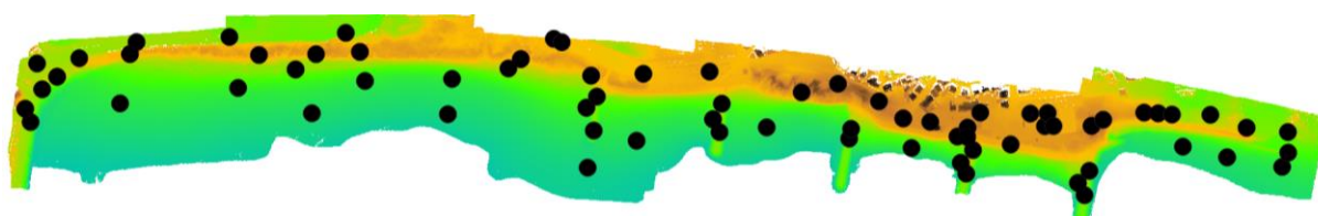
Figura 2.7 – Localização dos pontos coordenados em toda a extensão da praia
