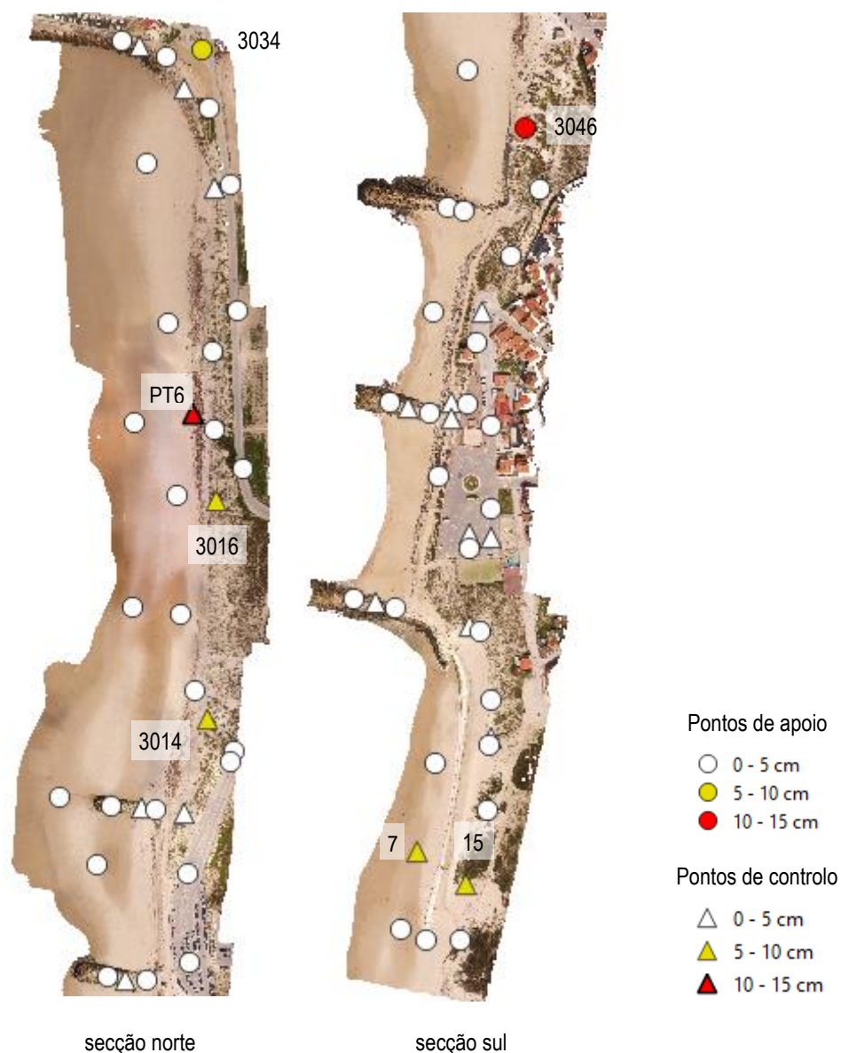
Figura 2.12 – Diferenças (distância) entre coordenadas GNSS e as obtidas do ortomosaico e da nuvem de pontos
