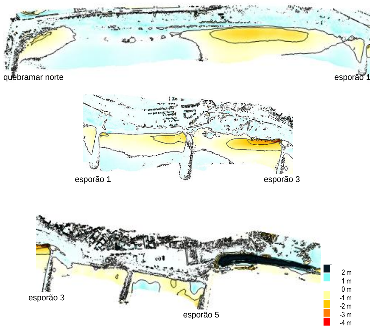
Figura 3.1 – Diferença entre modelos numéricos de superfície de 2019 e 2020 (equidistância de 1 m entre as isolinhas)
