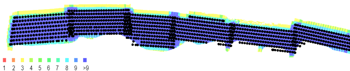
Figura 2.3 – Localizações da câmara fotográfica durante os voos (a cor de fundo indica o número de fotografias por pixel) em toda a extensão da praia
