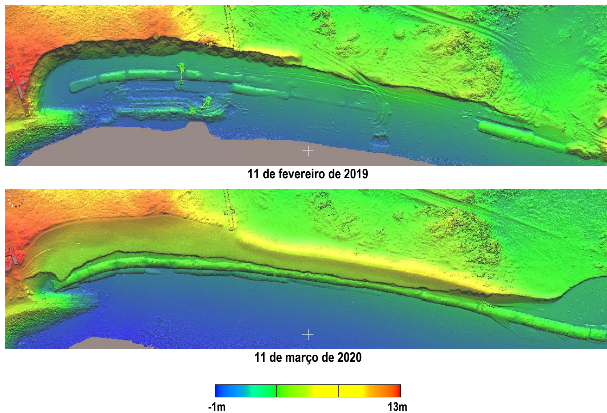
Figura 3.4 – Vista nadirais das nuvens de pontos de 2019 e 2020 da zona a sul do esporão 5 (coloração dependendo da altitude)
