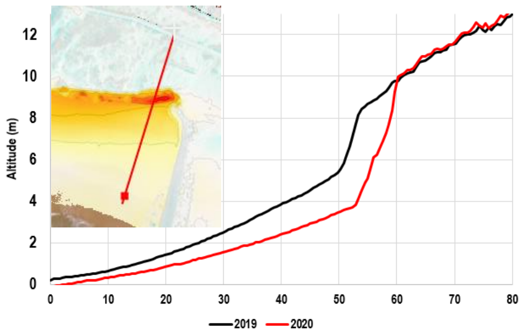
Figura 3.2 – Perfil da zona de maior alteração (erosão) da duna
